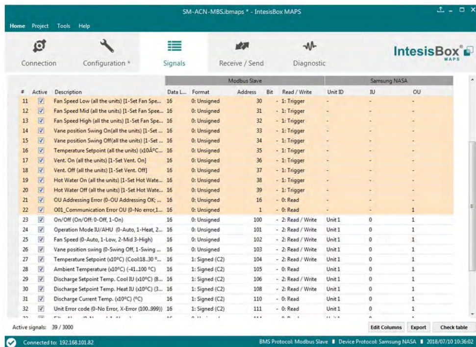
Abb. 4.8 IntesisBox MAPS Signale
