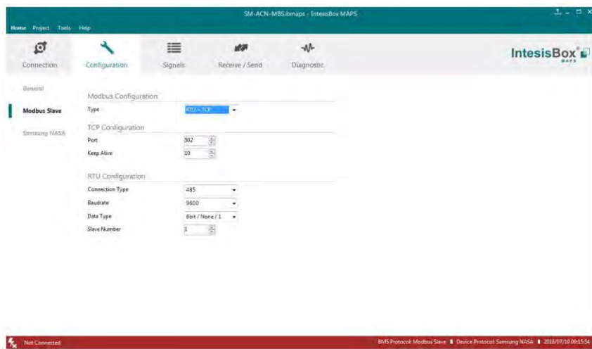
Abb. 4.3 IntesisBox MAPS Modbus Konfiguration
