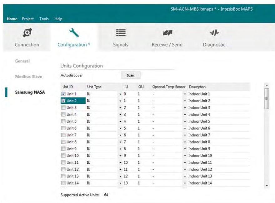
Abb. 4.4 IntesisBox MAPS Samsung NASA Konfiguration
