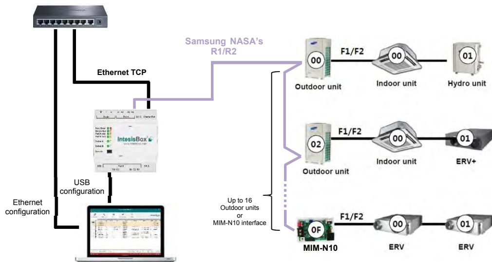
Integration eines Samsung NASA Systems in ein Modbus System
