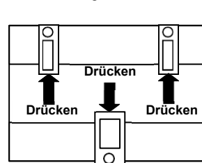
Befestigungsklammern in Standardposition (für DIN-Schienen-Montage)
